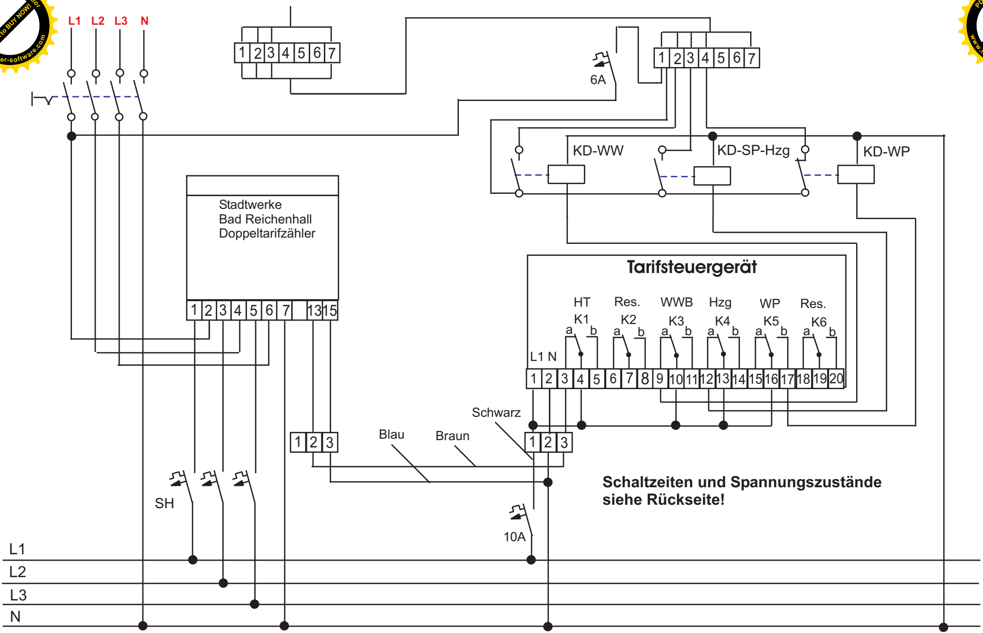
Anschlussbild Zähler mit Tarifsteuereinrichtung Grauer Rundsteuerempfänger
